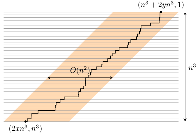
FIGURE 5. Limite d'échelle de B[(2xn^3, n^3) \rightarrow (n^3 + 2yn^3, 1)] .
